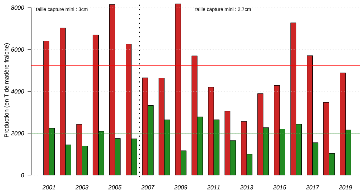
fig. 15 - Evolution de la production de coques en baie de Saint-Brieuc (de 1987 à 2019)
