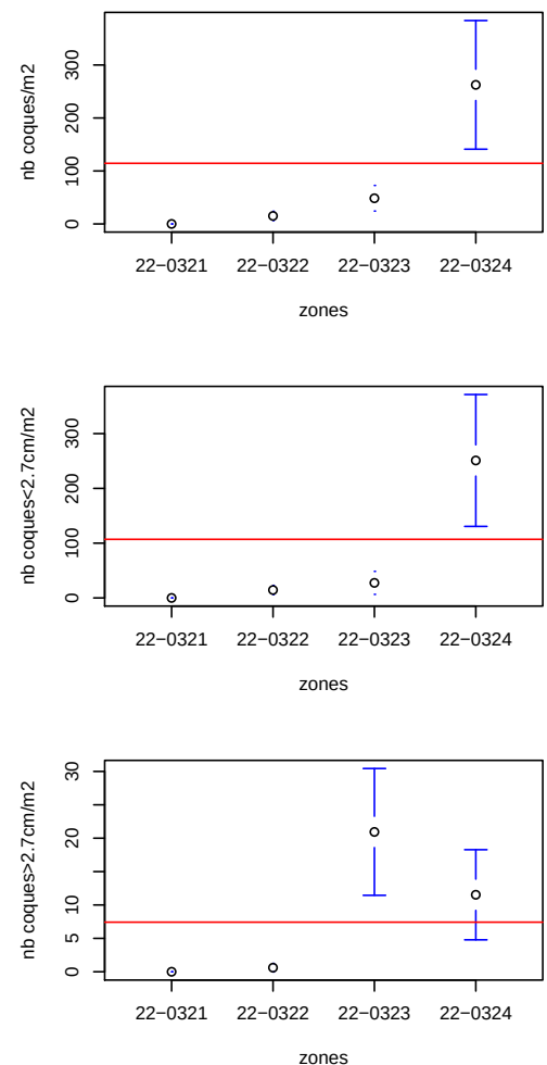
Fig. 3 - Nombres de coques par mètre carré observés en fonction des zones ( en rouge : valeur moyenne toutes zones confondues)
