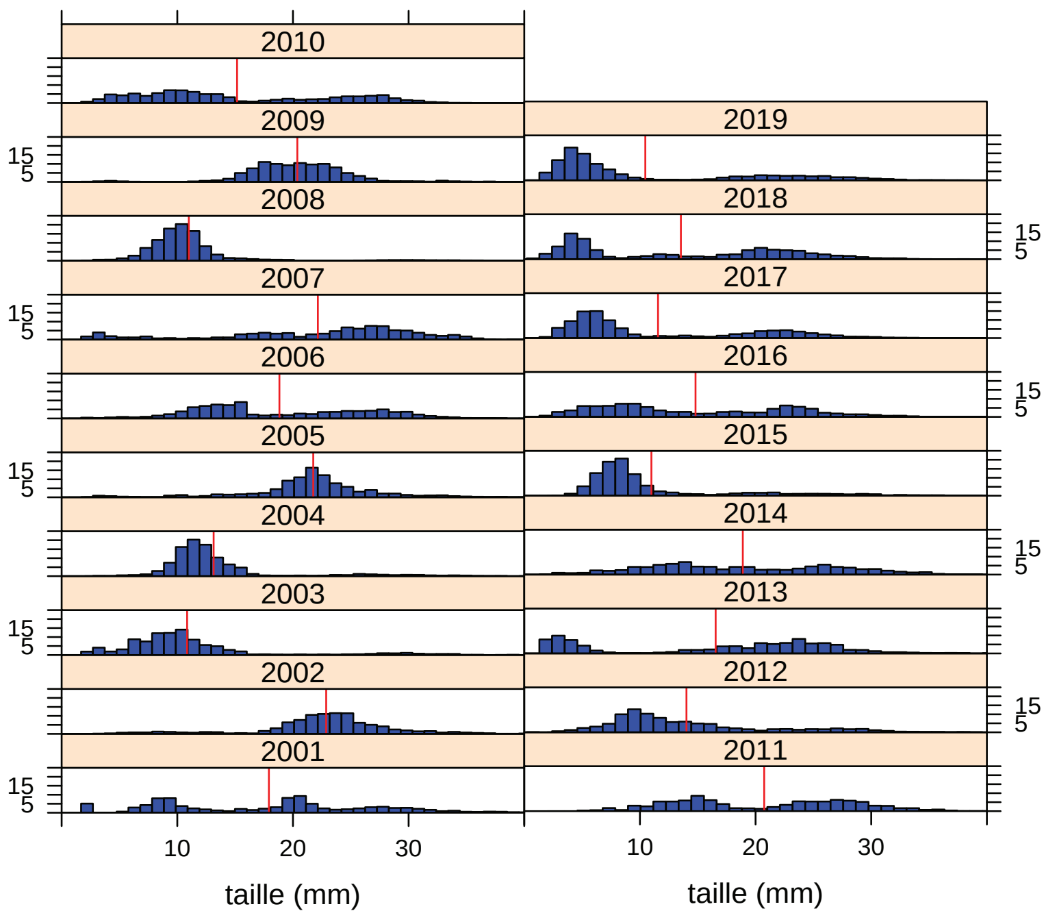
Fig 5c - Histogrammes en classe de taille du gisement observé entre 2001 et 2019.
