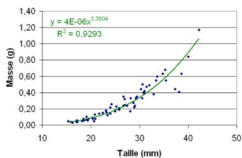
fig 12 - Relation entre la taille des coques (en mm) et leur masse (en g)
