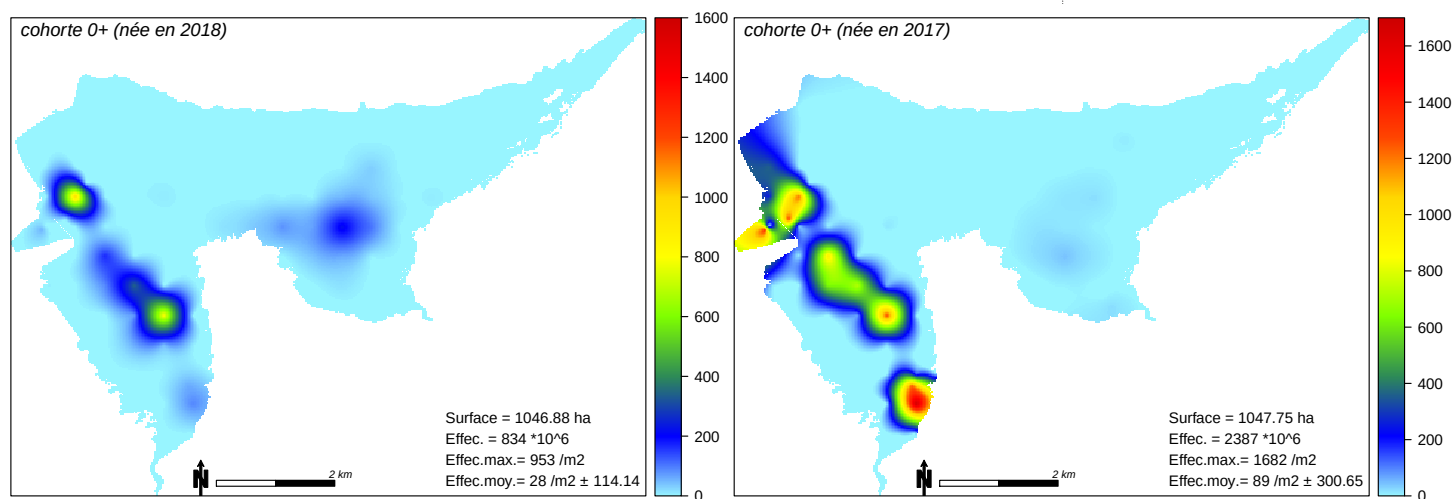
Figure 10b - Comparaison du recrutement observé en 2017 et en 2018
