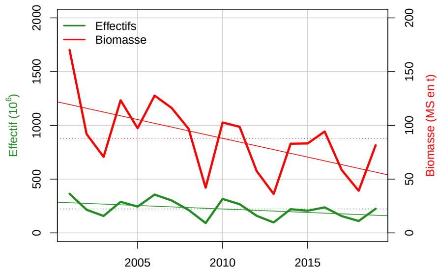
fig. 16 - Evolution des effectifs et de la biomasse de coque de plus de 2.7 cm (de 2001 à 2019). Afin de visualiser les évolutions du gisement, la modification de la taille légale de pêche (avant 2007) n'est pas pris en compte dans ce graphe.
