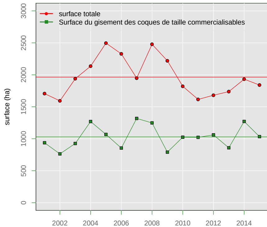
Fig 7 - Evolution des surfaces théoriques du gisement de coques calculées par modélisation (en hectares)
