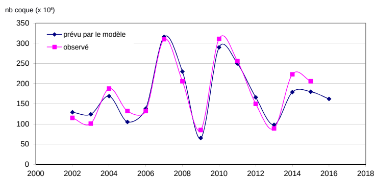
fig 14 - Evolution des effectifs de coques théoriques calculés par modélisation pour les coques de taille comercialisable prévu par le modèle (à l'année n-1) et observé à l'année n
