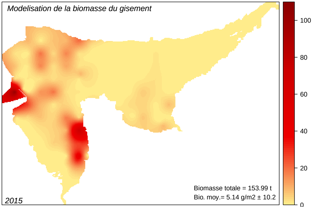
fig. 11 - Modélisation de la production du gisement de coques (en g.m -2 )
