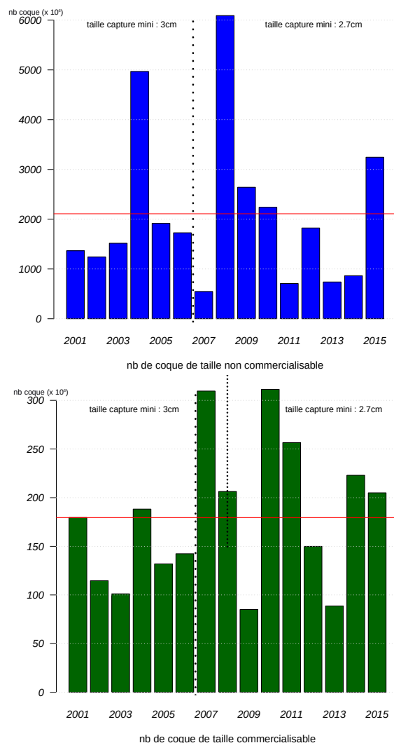
Tab 2 et fig 4 - Evolution des effectifs de coques théoriques calculés par modélisation pour l'ensemble du gisement (en millions de coques)
